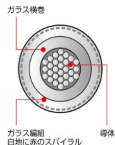
断面図
