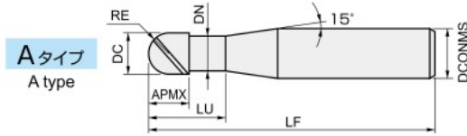
首下長5DCタイプ Under neck length 5DC type
