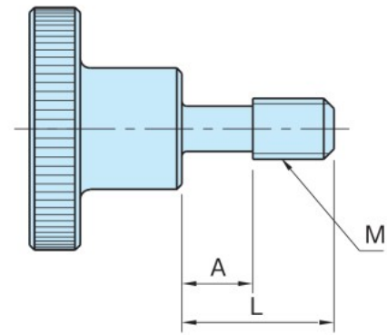
TKS-R-SUS (オネジ、脱落防止タイプ)
