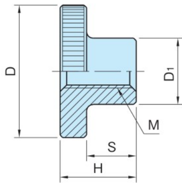
TKN TKN-SUS (メネジ貫通)
