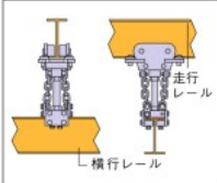
FRKS型 (固定支持ハンガー)
