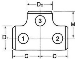
同径T T(S)
