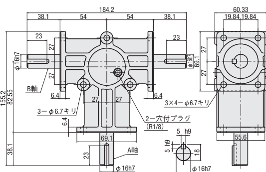
MMB2-T 質量/1.5kg 潤滑油脂量/15~35g
