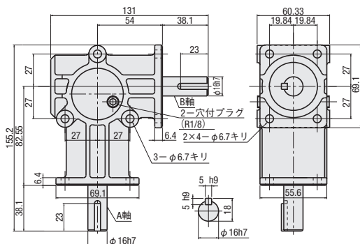
MMB2-D 質量/1.3kg 潤滑油脂量/15~35g
