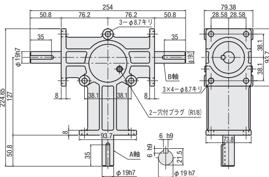
MMB3-T 質量/2.5kg 潤滑油脂量/40~70g
