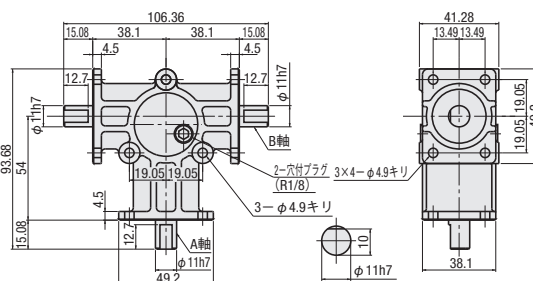
MMB1-T 質量/0.6kg 潤滑油脂量/5~15g
