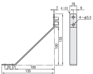
HPTGS5
