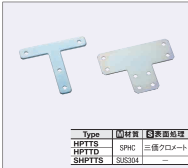
HPTTS5 SHPTTS5
