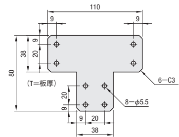
HPTTD5
