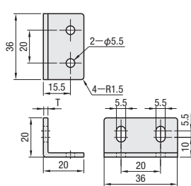
HPTGS5
