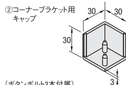
②コーナーブラケット用キャップ (ボタンボルト3本付属)
