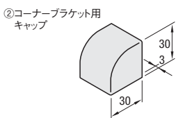
②コーナーブラケット用キャップ (六角穴付ボルト2本付属)
