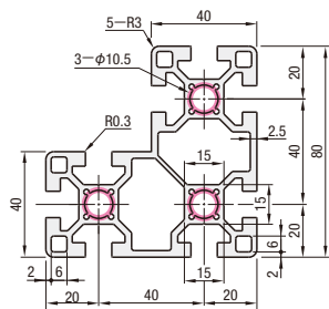
HFS8-808040
