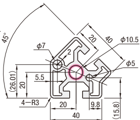
HFS8-808040
