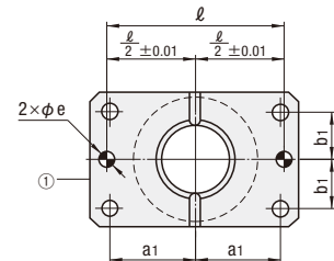
MYZP (ロック穴付・無給油)
