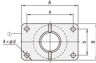
MY (給油)
