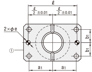
MYP (ロック穴付・給油)
