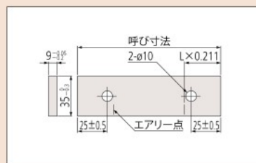
長尺ゲージブロック継ぎ足し穴の位置
