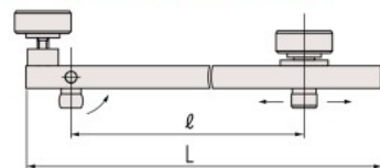
クランプコマ (2個) No.619036
