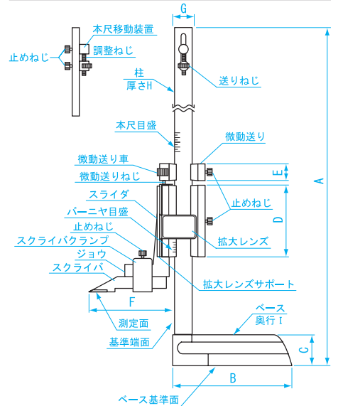
本尺目盛部 拡大レンズ (VHK-15)
