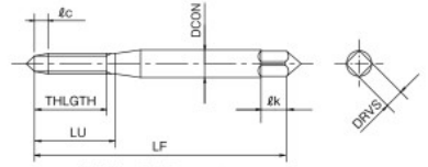
旧形状 Old Dimension
