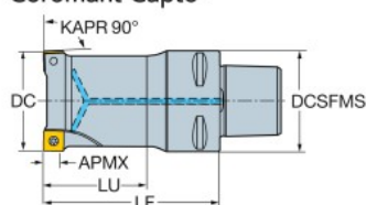
Coromant Capto®
