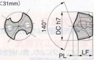
刃先交換ヘッド MTL 型 刃径φ12.0~17.3mm 寸法(mm)
