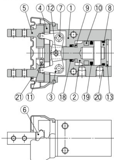
複動形/フィンガ閉状態
