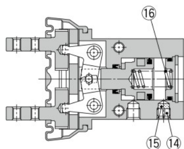
単動形/常時開形
