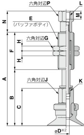
構造図 P.118 バッファAss'y P.124
