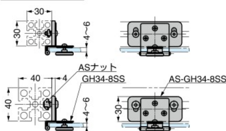
取付寸法図
