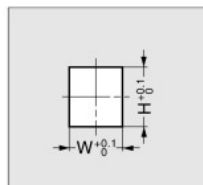
取付穴加工図
