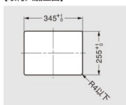
【取付穴加工図】
