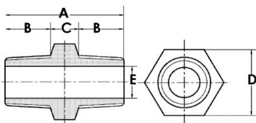
六角ニップル
