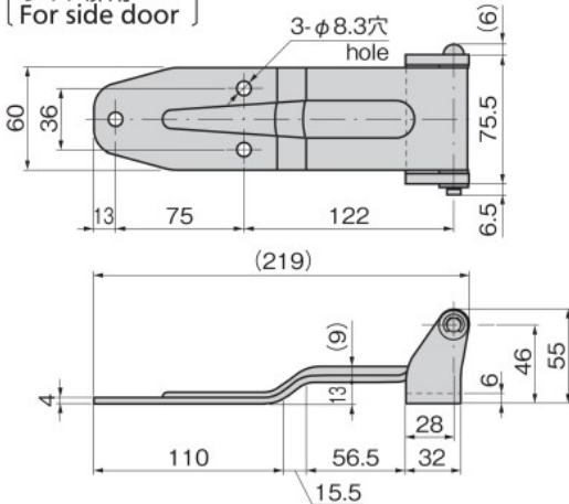
[FB-812-1-L サイド扉用 For side door]
