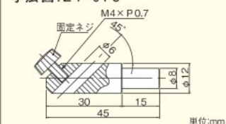
寸法図:ZY-073
