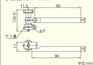
寸法図:ZY-073
