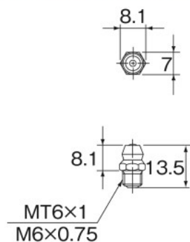
A-MT6×1形 (MT6×1) A-M6F形 (M6×0.75)
