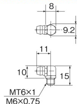
C-MT6×1形 (MT6×1) C-M6F形 (M6×0.75)
