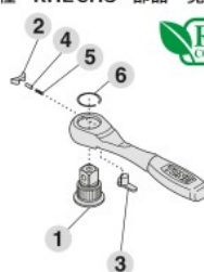
RH2CHS 部品展開図
