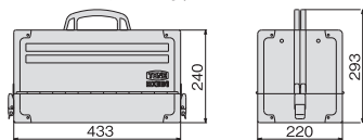
■ BX331 ケース寸法
