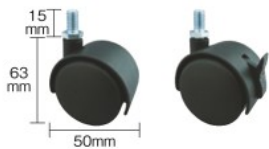
TDG-50-M8 (自在) TDGS-50-M8 (自在ストッパー付き) (ねじ込み式双輪キャスター)
