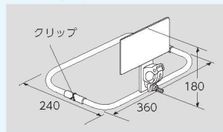
■ 寸法図 (mm)
