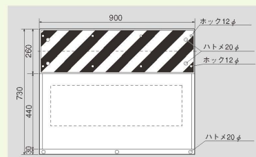
■ 寸法図 (mm)
