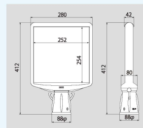
■寸法図(mm)
