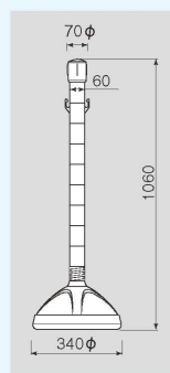
■寸法図(mm)
