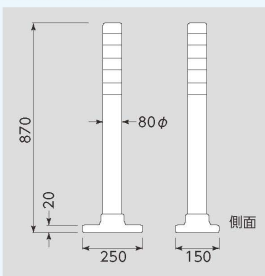
■寸法図(mm)
