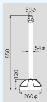
■寸法図(mm)
