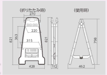
■寸法図 (mm)
