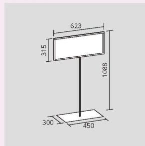
■ 寸法図 (mm)
