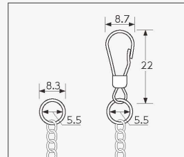
寸法図(mm)
