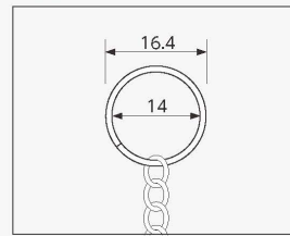
寸法図(mm)
