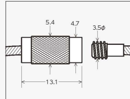
寸法図(mm)
