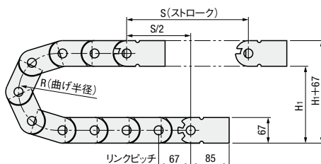
取付関係図
