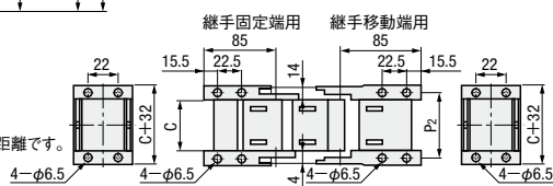
取付関係図
