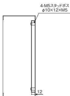
B-B断面
