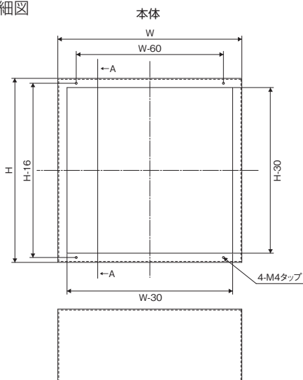
詳細図
